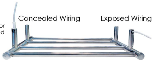
Universal Wiring Options
